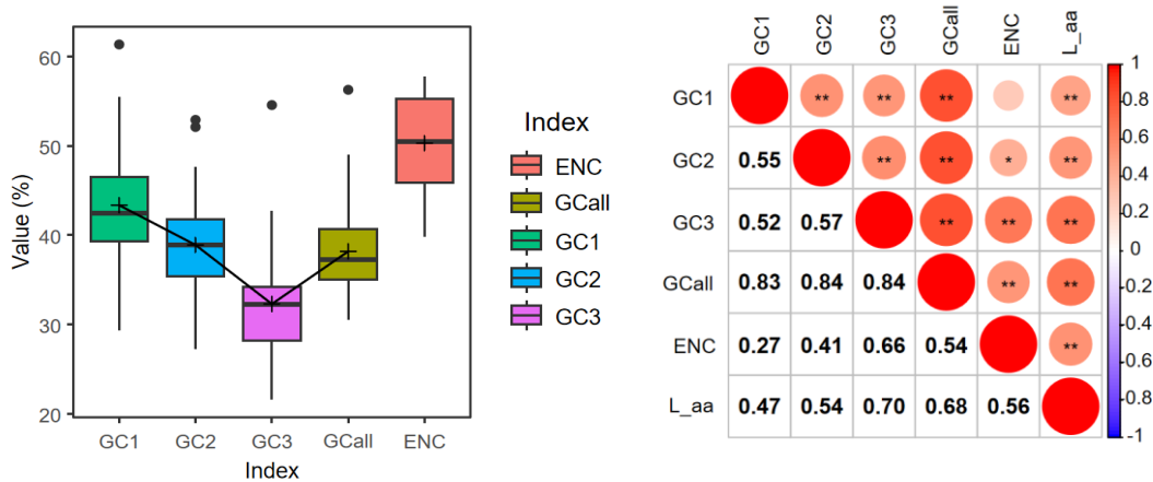
a) GC1、GC2、GC3、GC1+2+3 和 ENC 的分布, 平均值的位置用“+”表示 b) 紫叶苔线粒体基因组密码子偏好主要指标的相关性分析
