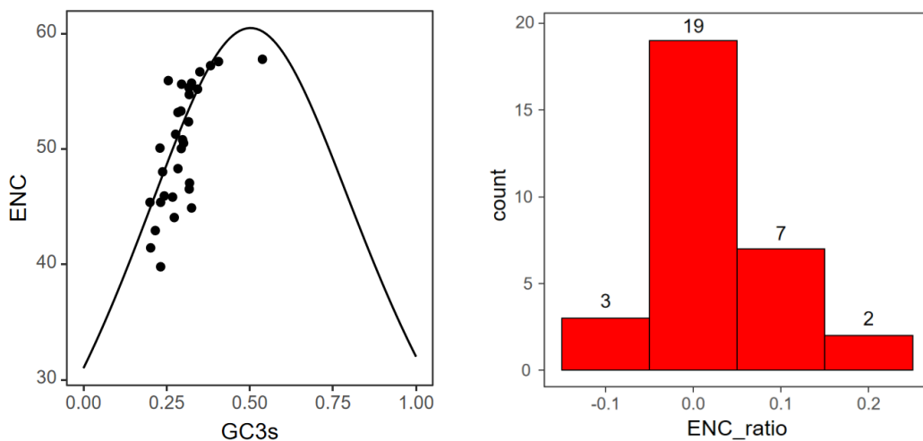
a)紫叶苔线粒体基因组的 ENC-plot 分析
