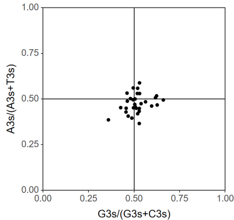
图 5 紫叶苔线粒体基因组的 PR2-plot 分析
